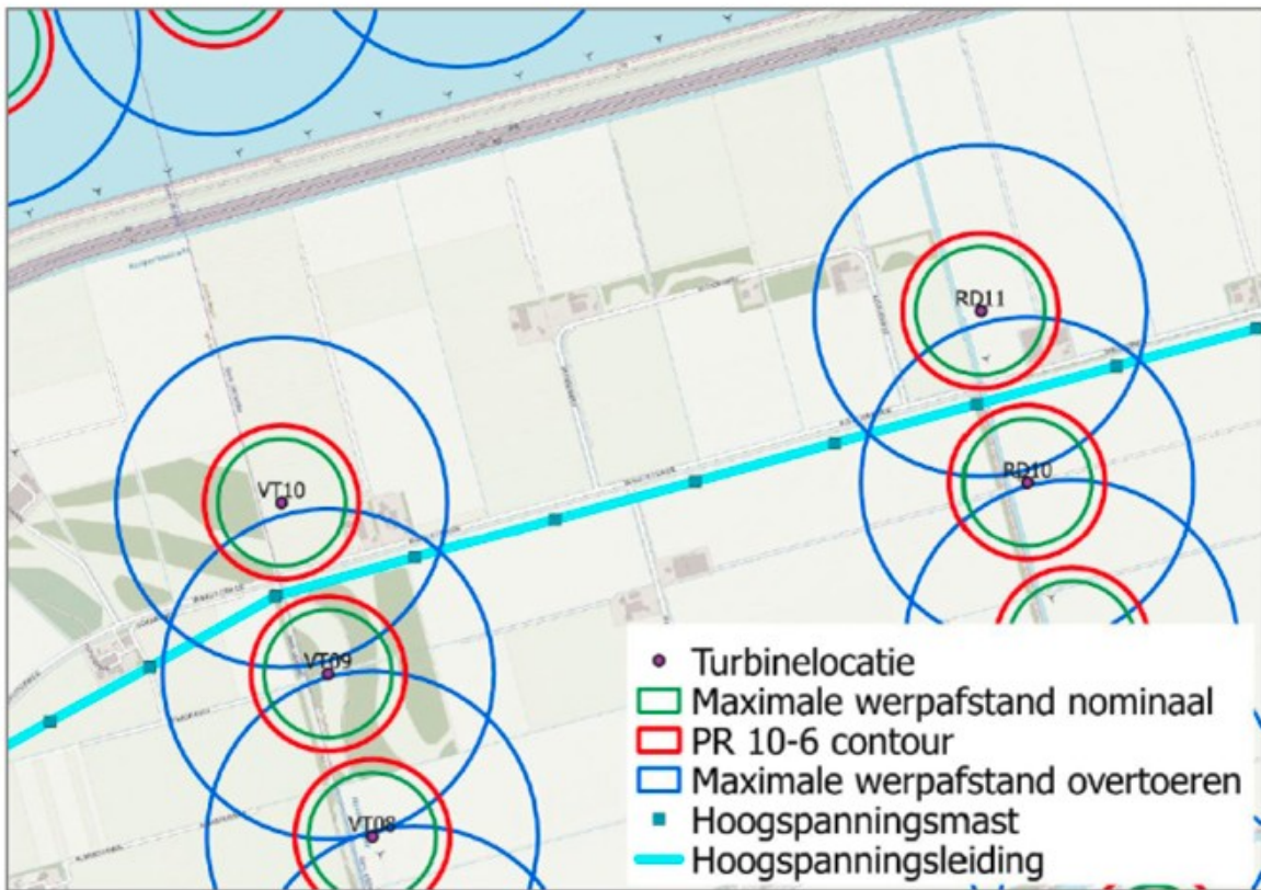
Figuur 13. Hoogspanningsmasten en -leidingen binnen maximale werpafstand
